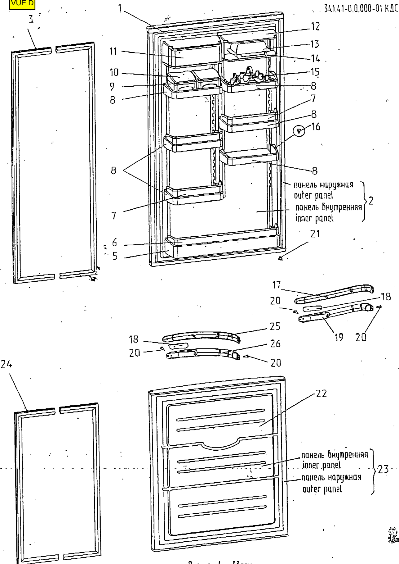
Рисунок 4 - Двери
